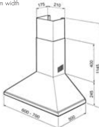
KSED72X 70cm width
